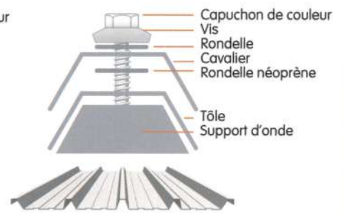
Schema de fixation sommet d'onde sur tôle 1000P
