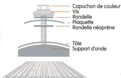
Schema de fixation sommet d'onde sur tôle ondulée
